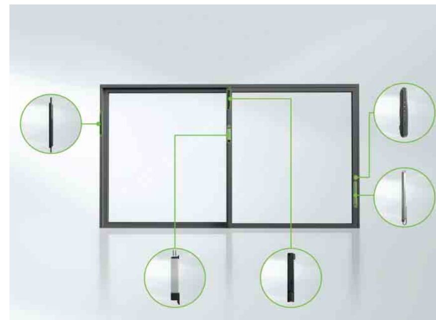
Detaildarstellung der vollintegrierten mechatronischen Beschlagkomponenten Detailed illustration of the fully integrated mechatronic fittings components
